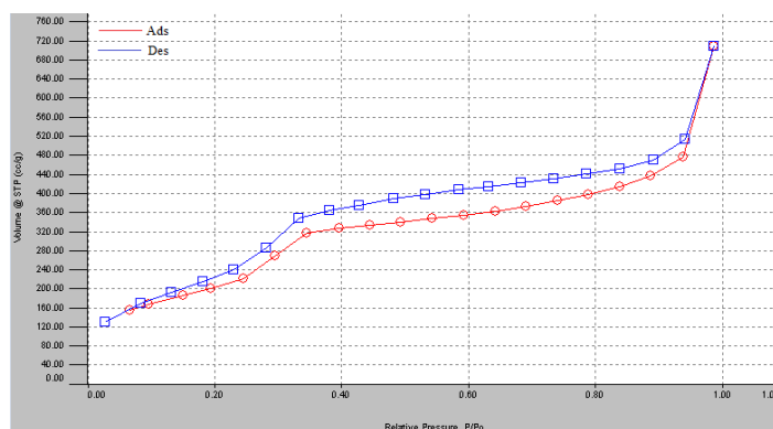
Figura 5. Isotermas de adsorción-desorción de N_2 de las partículas sintetizadas.
