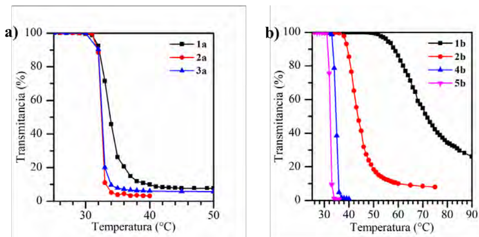
Fig. 3. Estudio de propiedades termosensibles de los copolímeros (PHEA- b -PNIPAM) 6 en agua mediante UV-Vis.
