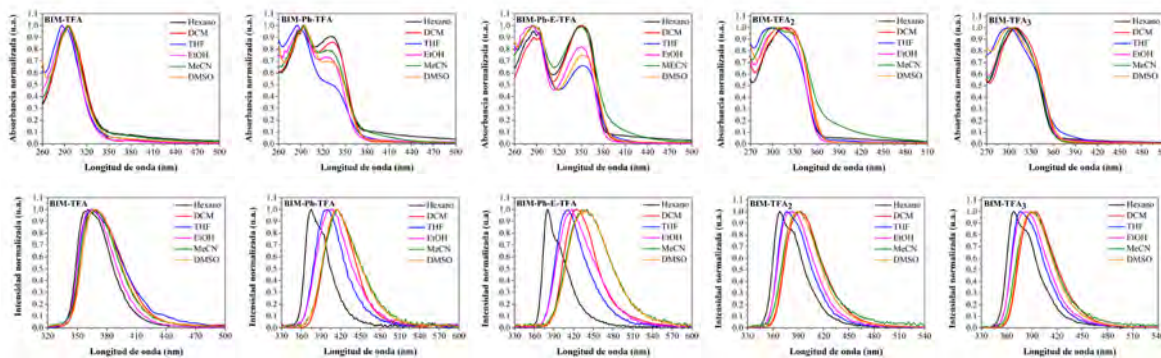
Fig. 3. Espectros de absorción (arriba) y fluorescencia (abajo) de los derivados 2,2'-BIM-TFA en disolventes de diferente polaridad a 10 \mu\text{M} .
