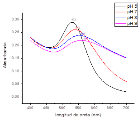
Fig. 2. Espectros UV-Vis de las disoluciones de AuNPs obtenidas con extracto de Eucalyptus globulus a diferentes pHs.
