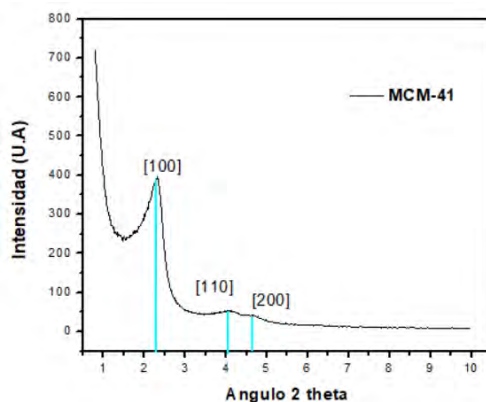
Fig. 4. Difractograma del resultado de análisis SAXRD de las partículas sintetizadas con silicato de sodio.
