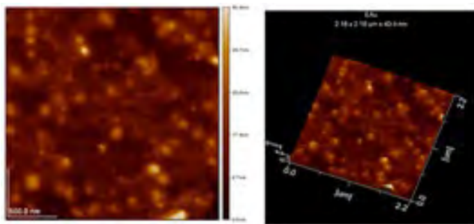
Fig. 3. Imágenes AFM topográfica (2.18 \mu\text{m} x 2.18 \mu\text{m} x 43.4 nm) en modo "shaded" de las nanopartículas de oro obtenidas a pH = 8.
