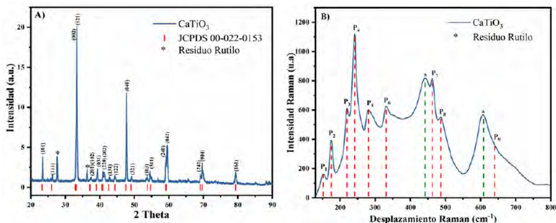
Fig. 2. Espectros de las partículas de \text{CaTiO}_3 sintetizadas con sistema ortorrómbico: (A) Difractograma y (B) espectro Raman.
