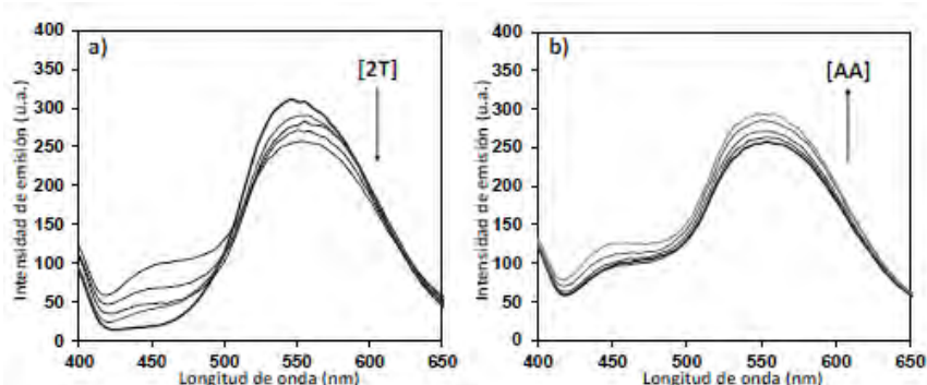
Fig. 3. Espectros de emisión de nanopartículas de \text{AgInS}_2/\text{ZnS} en presencia de 2-tionaftol (0-30 \mu\text{M} )(a). Espectros de emisión de nanopartículas de \text{AgInS}_2/\text{ZnS} -2-Tionaftol y acrilamida (5-30 \mu\text{g L}^{-1} ) (b).
