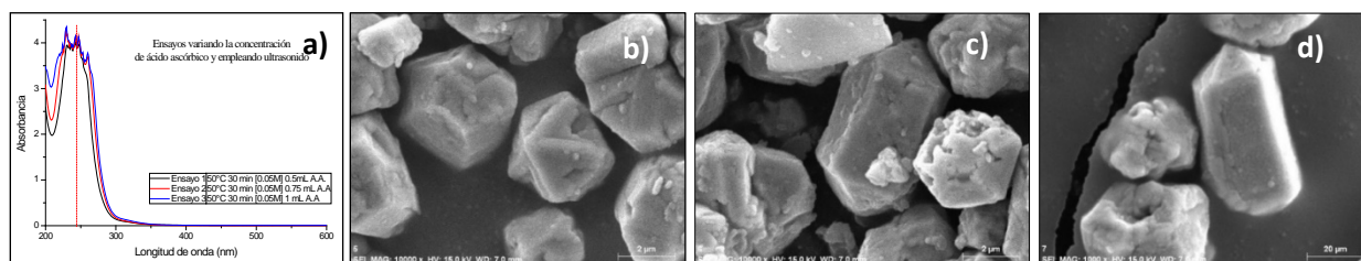
Fig. 1. (a) Absorción máxima UV-Vis de los MCs en 245 nm, microestructura de los MCs empleando: (b) 0.5 mL de AA (c) 0.75 mL de AA y (d) 1 mL de AA.
