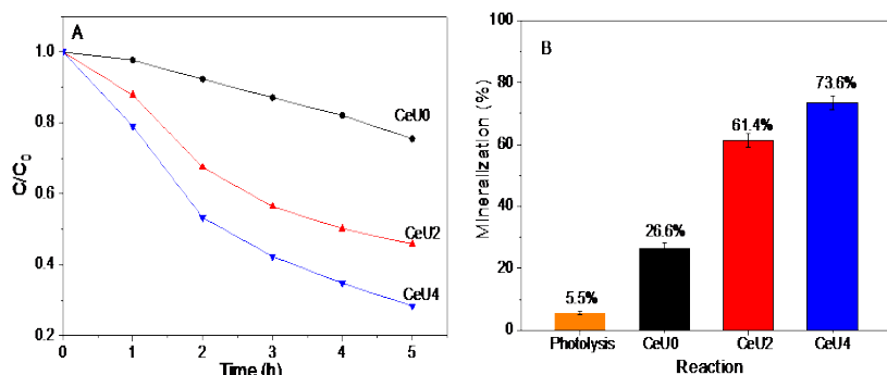
Fig. 3. (A) Concentración relativa de 3-clorofenol durante el proceso fotocatalítico y (B) porcentaje de eliminación de 3-clorofenol determinado por COT a la quinta hora de reacción.
