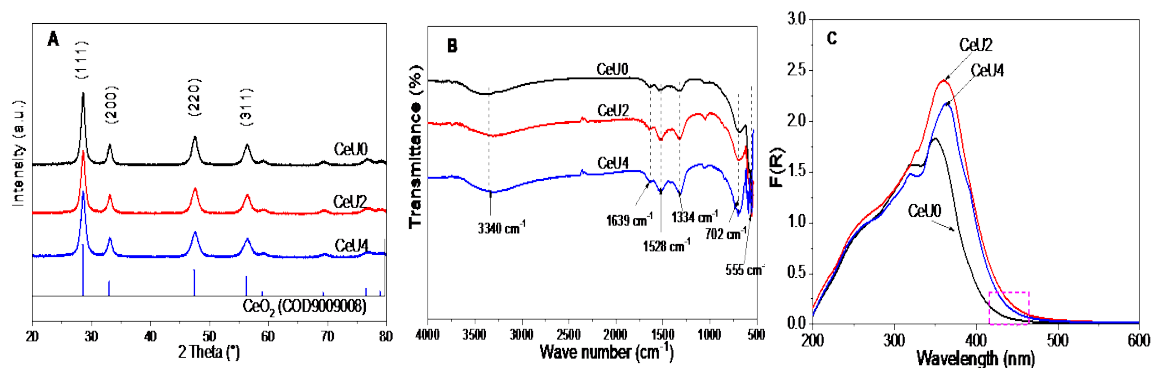
Fig. 1. (A) Difractogramas de rayos X, (B) espectros FT-IR y (C) Función Kubelka-Munk de los CeO 2 sintetizados.
