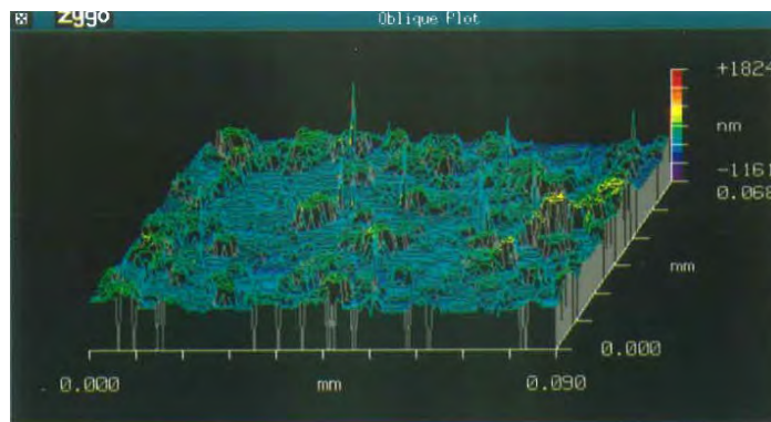
Fig. 1. Imagen de microscopia interferométrica en la que se observan una matriz de Ni-P-2% Al 2 O 3 , sin tratamiento térmico, de morfología "esférica" en forma de "islas". MI. 40X R a promedio 1.542 µm.
