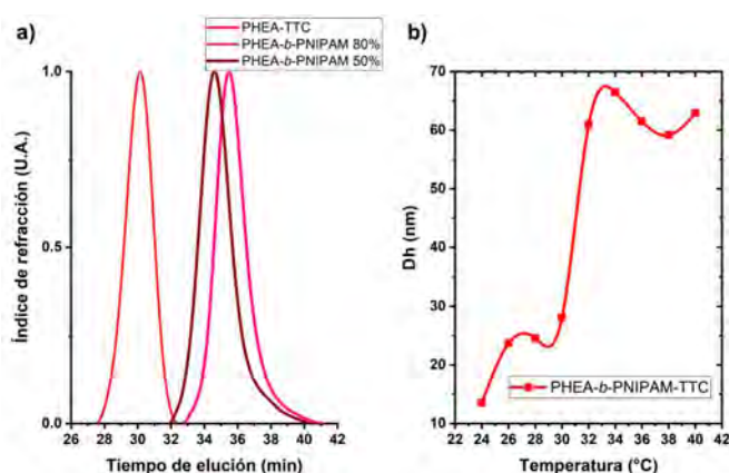
Fig. 1. Resultados del copolímero PHEA- b -PNIPAM. (a) cromatograma de GPC para PHEA- b -PNIPAM con NIPAM en un porcentaje de 80 % y 50 % (b) y de DLS.
