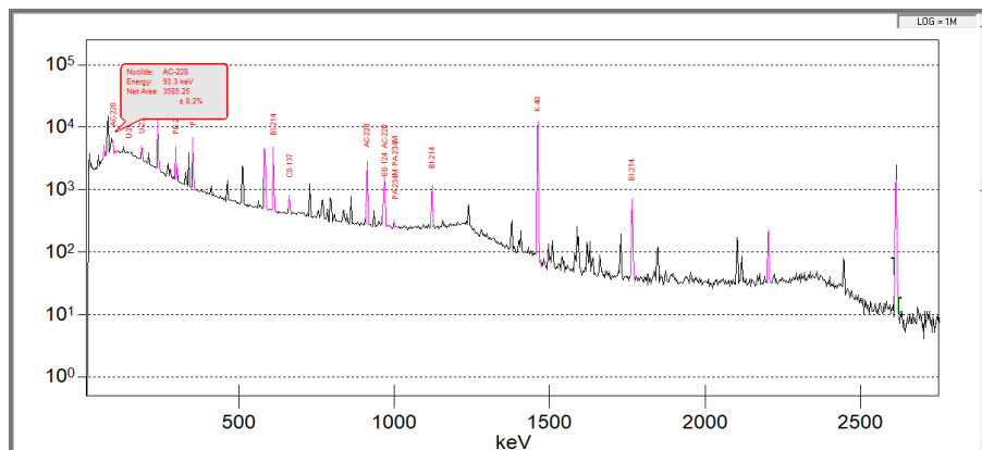
Fig. 5. Espectro gamma característico de las muestras.
