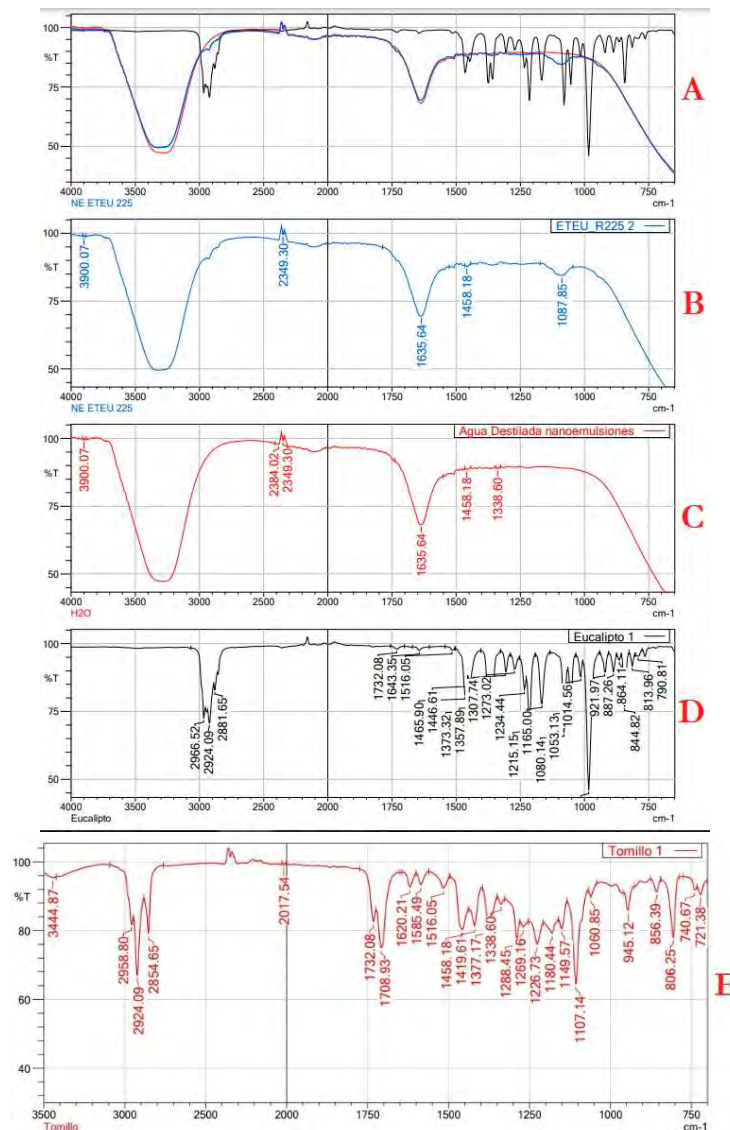
Fig. 3. Espectros IR de las muestras analizadas (A) sobreposición de espectros de agua destilada, aceite esencial de eucalipto, NE ETEU, (B) NE ETEU, (C) Agua destilada, (D) Aceite esencial de eucalipto, y (E) Aceite esencial de tomillo.
