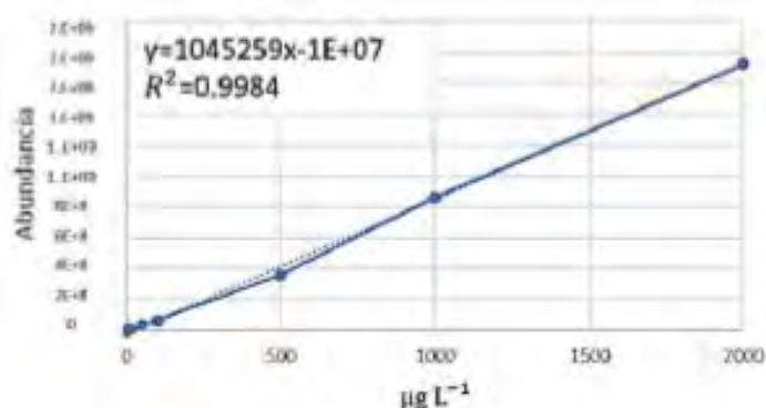
Fig. 4. Curva de calibración del diclofenaco por GC-MS.
