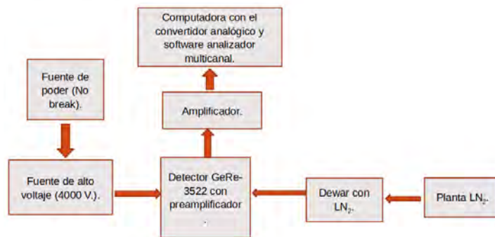
Fig. 4. Diagrama del sistema de espectrometría gamma.
