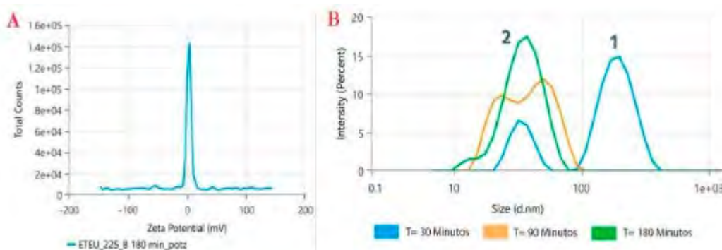
Fig. 1. (A) Gráfica de distribución de potencial Z muestra 180 minutos de baño ultrasónico (0.6573 mV), (B) Gráfica de análisis de distribución de tamaños a diferentes tiempos de sonicación de baja energía.
