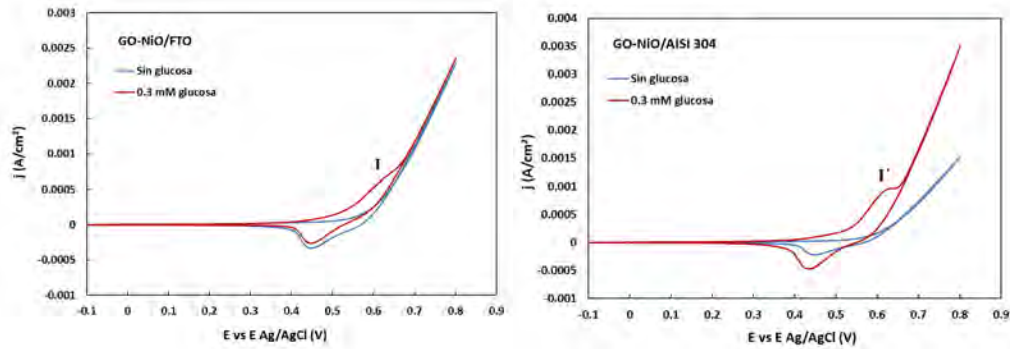
Fig. 2. Respuesta electroquímica de los electrodos en 0.1 M KOH en ausencia y presencia de 0.3 mM de glucosa (a) Electrodo GO-NiO/FTO (b) Electrodo GO-NiO/AISI 304.
