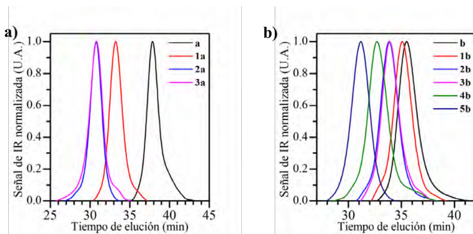
Fig. 2. Cromatograma de GPC en fase móvil de THF a 35 °C de extensión de cadena de NIPAM utilizando (a) (PHEA 5 ) 6 y (b) (PHEA 20 ) 6 como macroagente RAFT.
