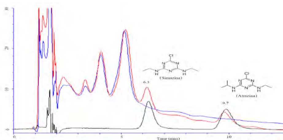
Fig. 2. Cromatograma de muestra fortificada con atrazina y simazina 0.4 µg (en rojo), muestra blanca (en azul) y estándar a 4 ppm (en negro).
