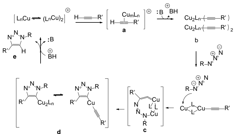
Fig. 3. Cicladición de azidas y alquinos terminales catalizada por Cu(I).
