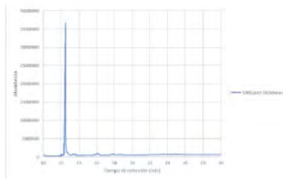
Fig. 3. Cromatograma del diclofenaco por GC-MS.
