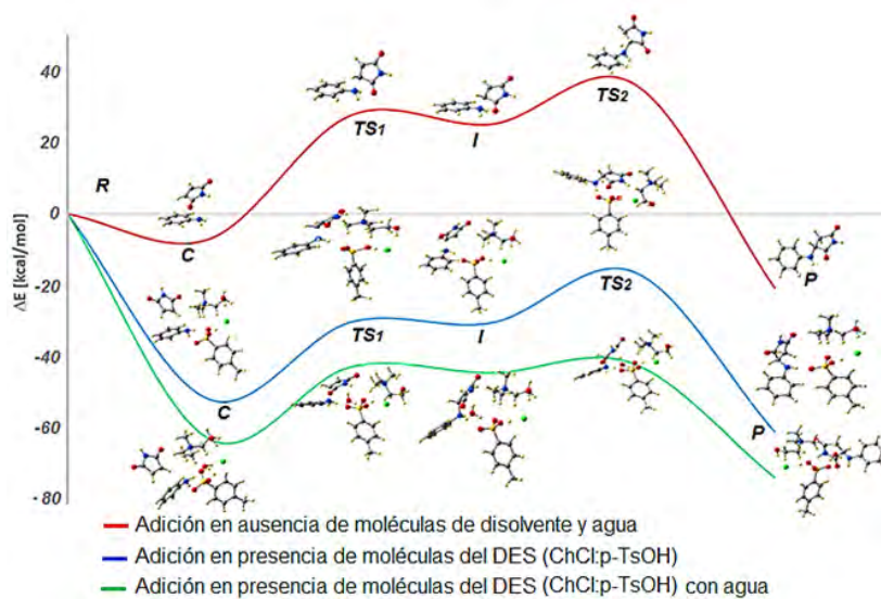
Fig. 1. Perfiles de energía para la reacción de adición.
