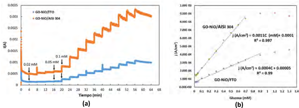
Fig. 3. Resultados de las pruebas de sensado electroquímico de glucosa de los electrodos GO-NiO/FTO y GO-NiO/AISI 304 (a) Cronoamperometrías (b) Cuantificación de glucosa.
