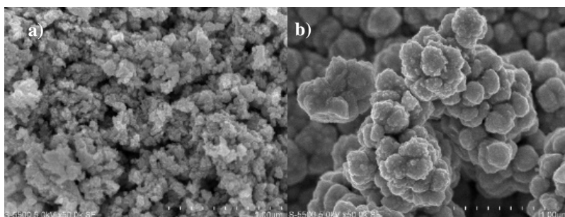
Fig. 2. (a) Muestra MC1, (b) muestra MS1.
