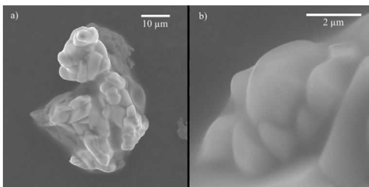
Fig. 1. Micrográficas MEB de titanita, (a) 3.23 kx, (b) 30.8 kx.
